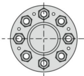
„C“ centerline mount
